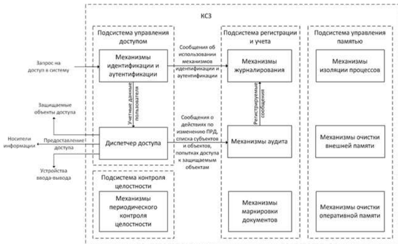
Рис. 1 – Логические компоненты КСЗ
