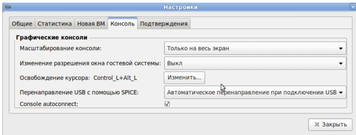
Рис. 14 – Вкладка «Консоль»
