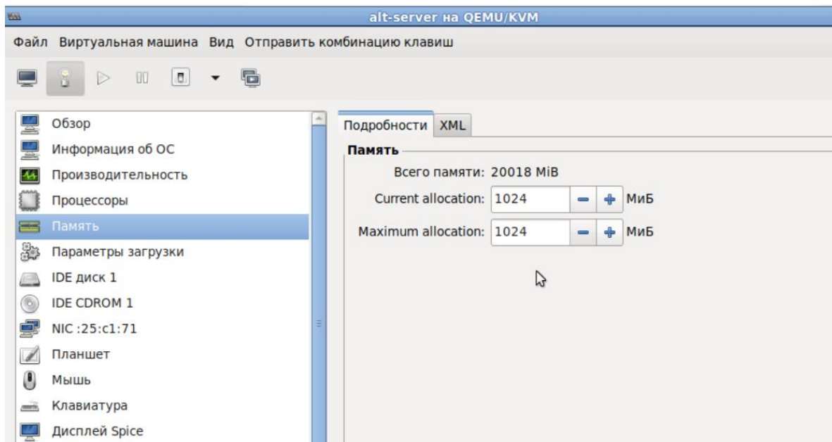
Рис. 11 – Вкладка «Память»
