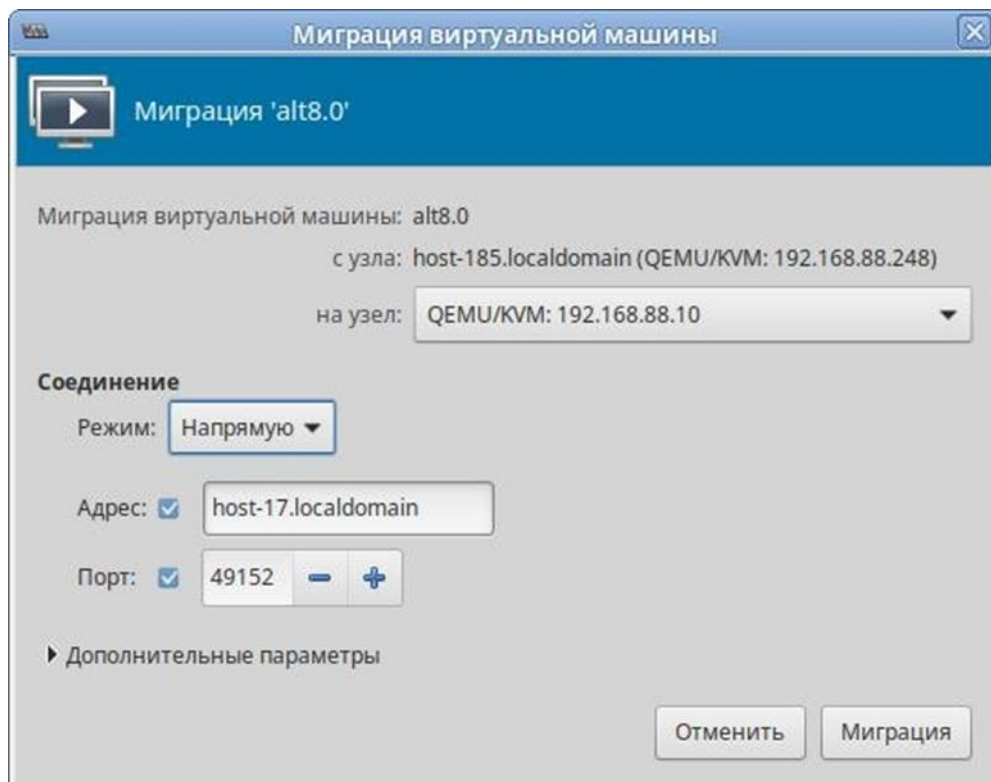
Рис. 26 – Миграция ВМ
