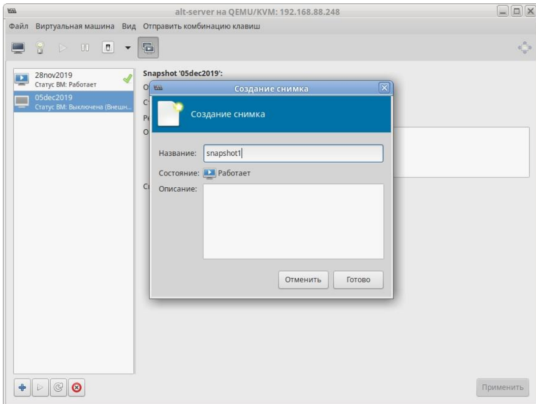
Рис. 28 – Создание снимка
