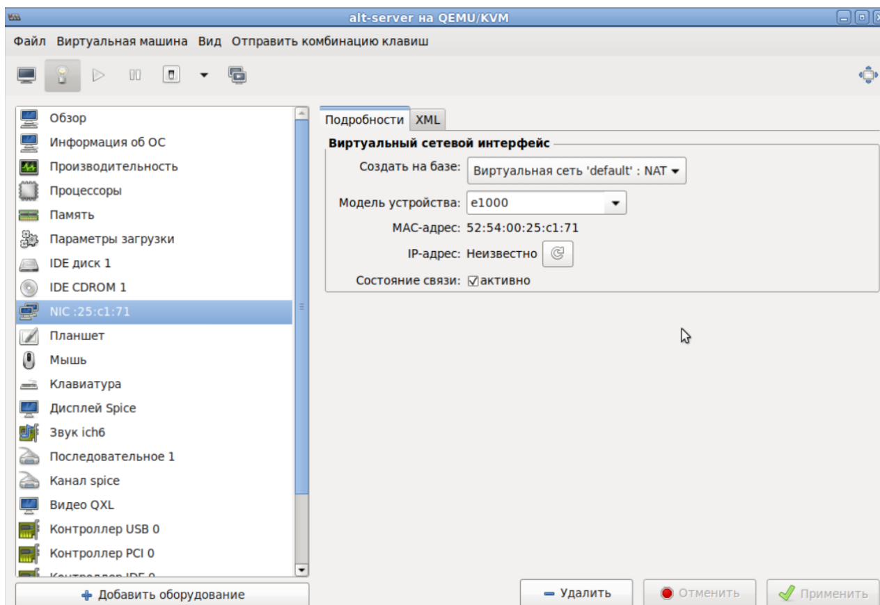
Рис. 12 – Вкладка «Сеть»
