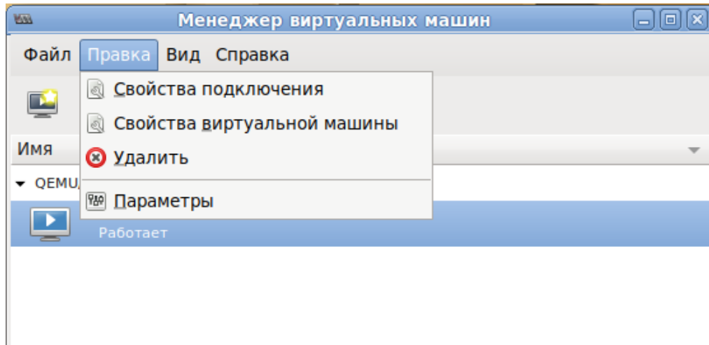
Рис. 15 – Меню «Правка»
