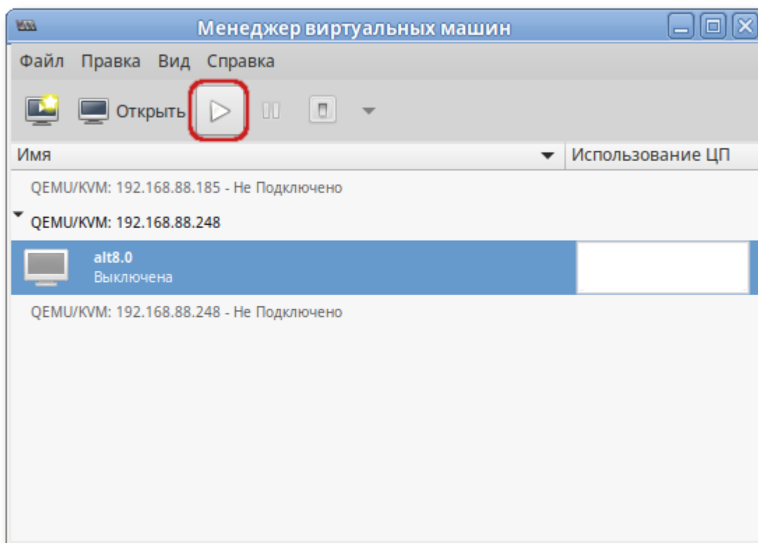
Рис. 22 – Включение VM
