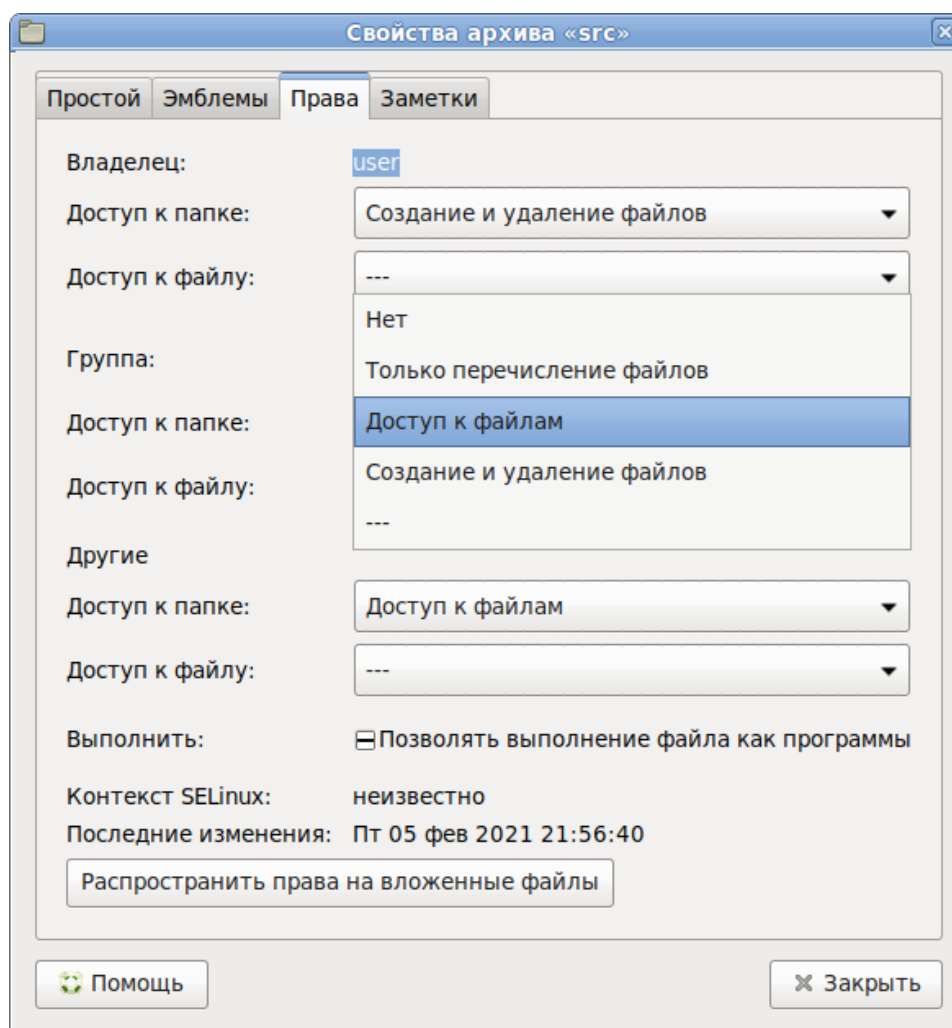
Рис. 12 – Изменение прав доступа на папку в файловом менеджере Caja
