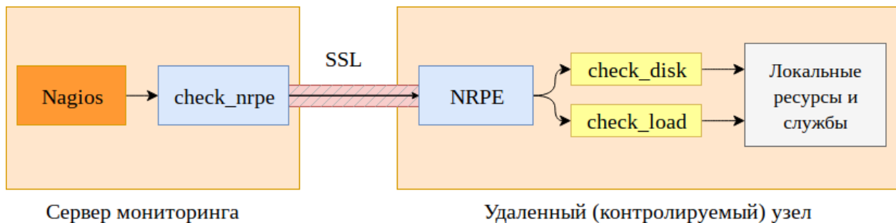
Рис. 86 – Взаимодействие сервера мониторинга с удаленным узлом
