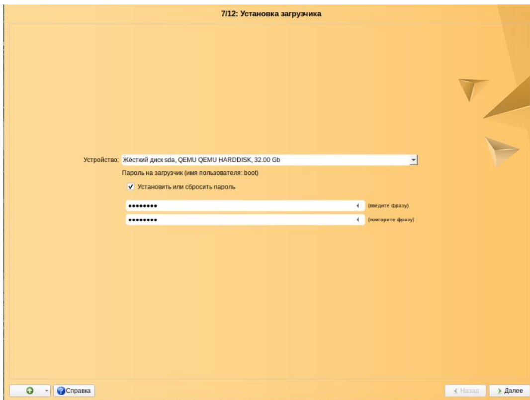
Рис. 21 – Установка загрузчика
