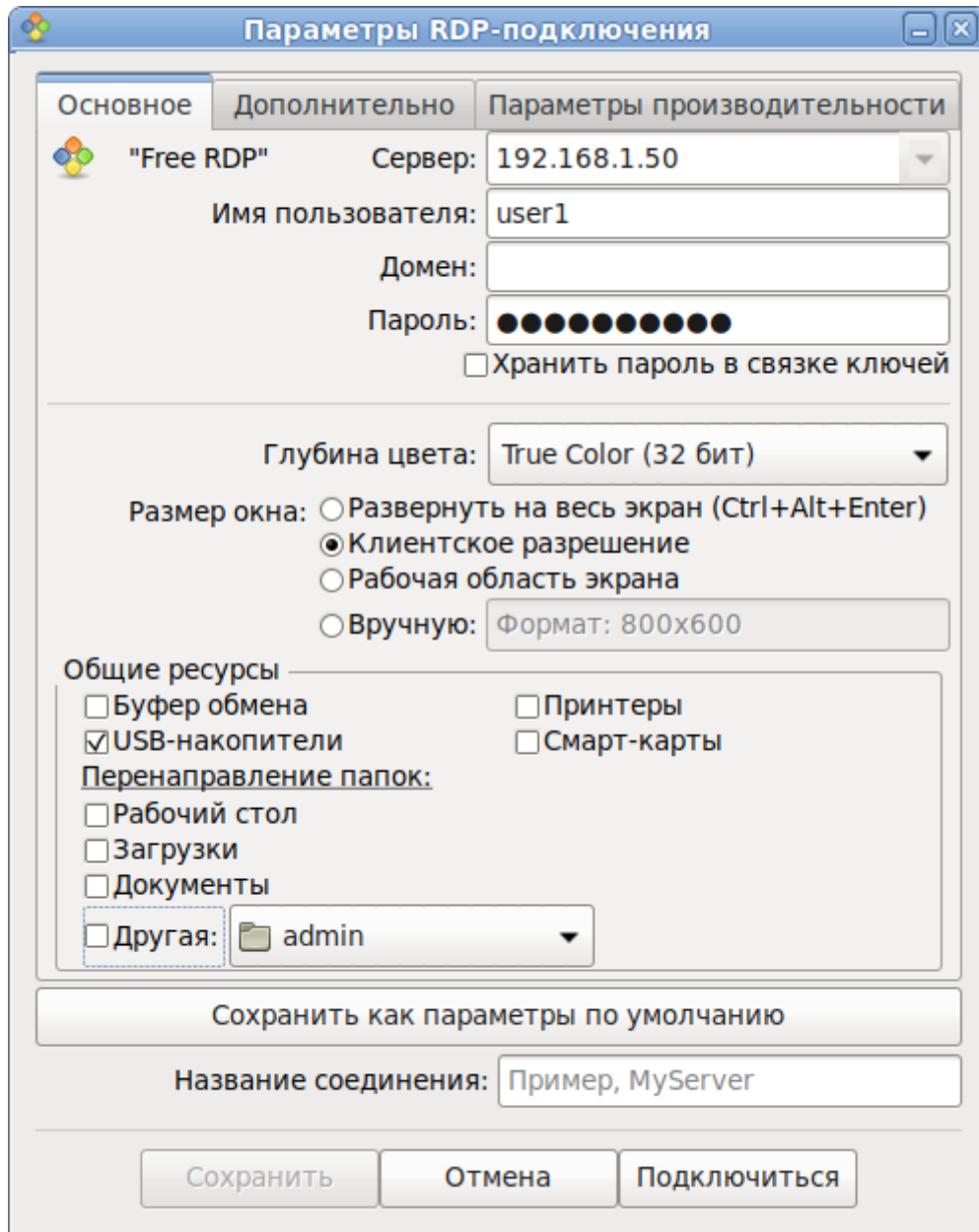
Рис. 209 – Настройки RDP-подключения
