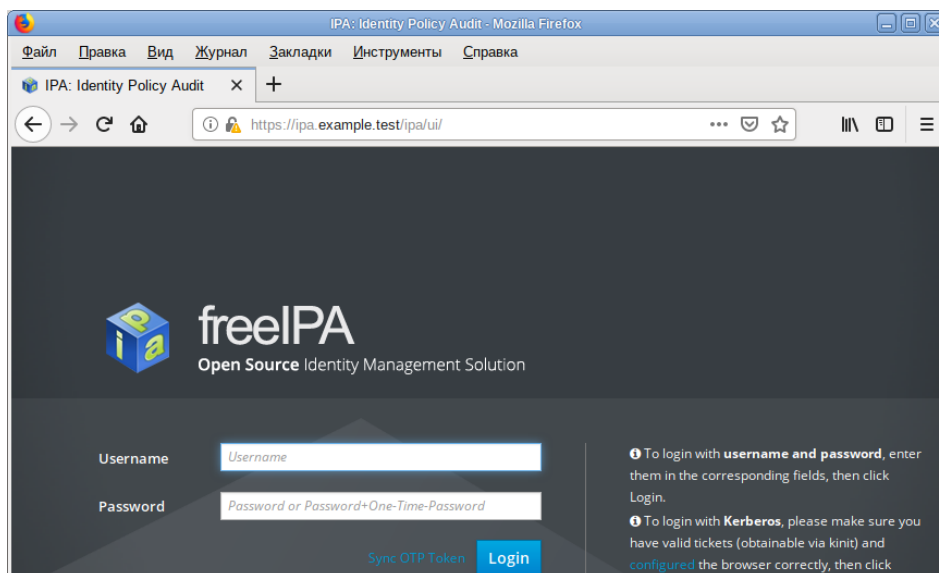
Рис. 170 – Веб-интерфейс FreeIPA
