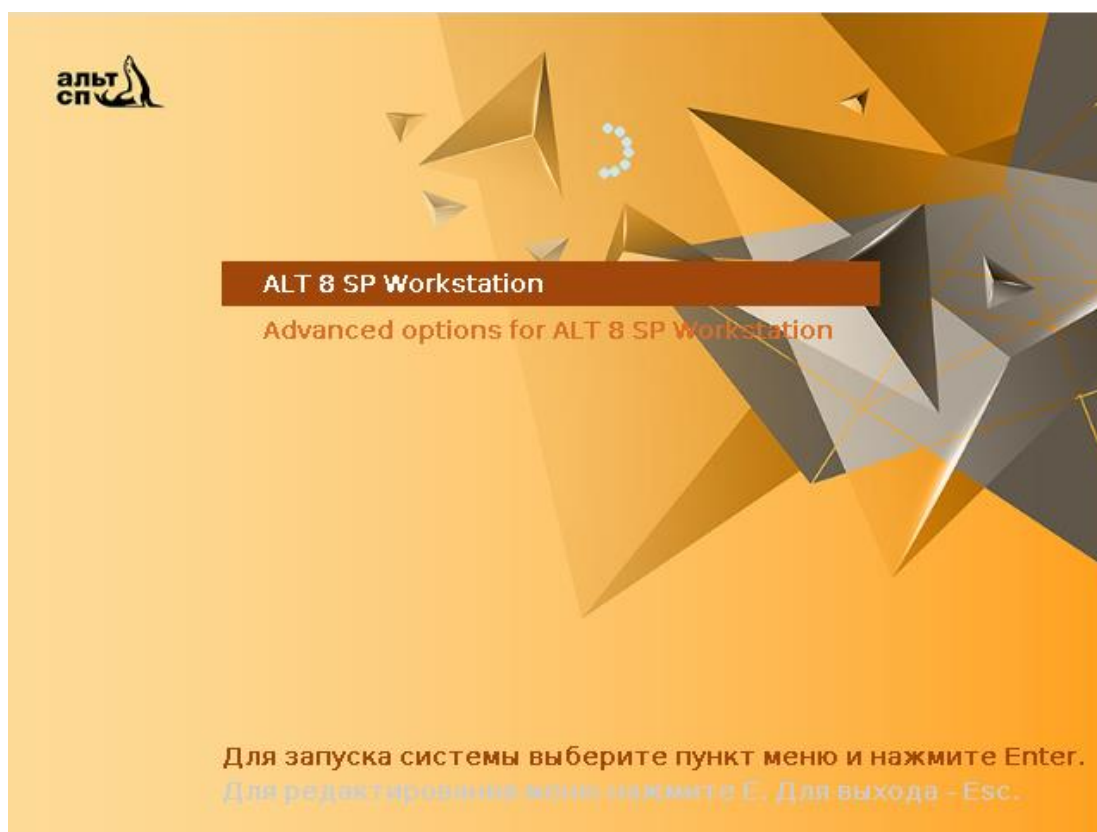
Рис. 58 – Варианты загрузки
