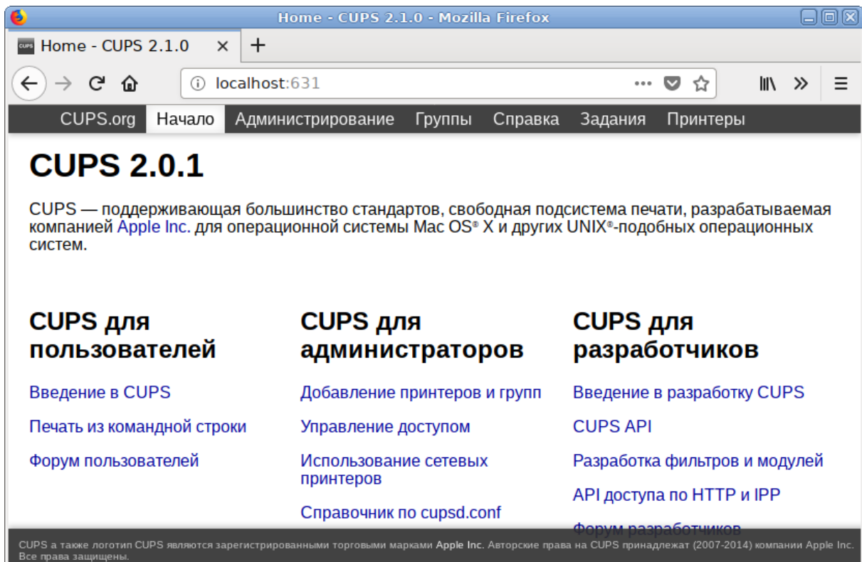
Рис. 198 – Веб-интерфейс CUPS
