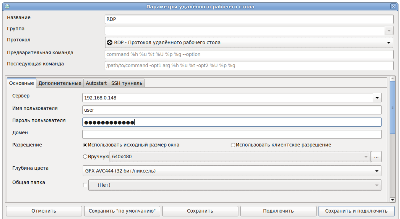
Рис. 206 – Настройки RDP-подключения
