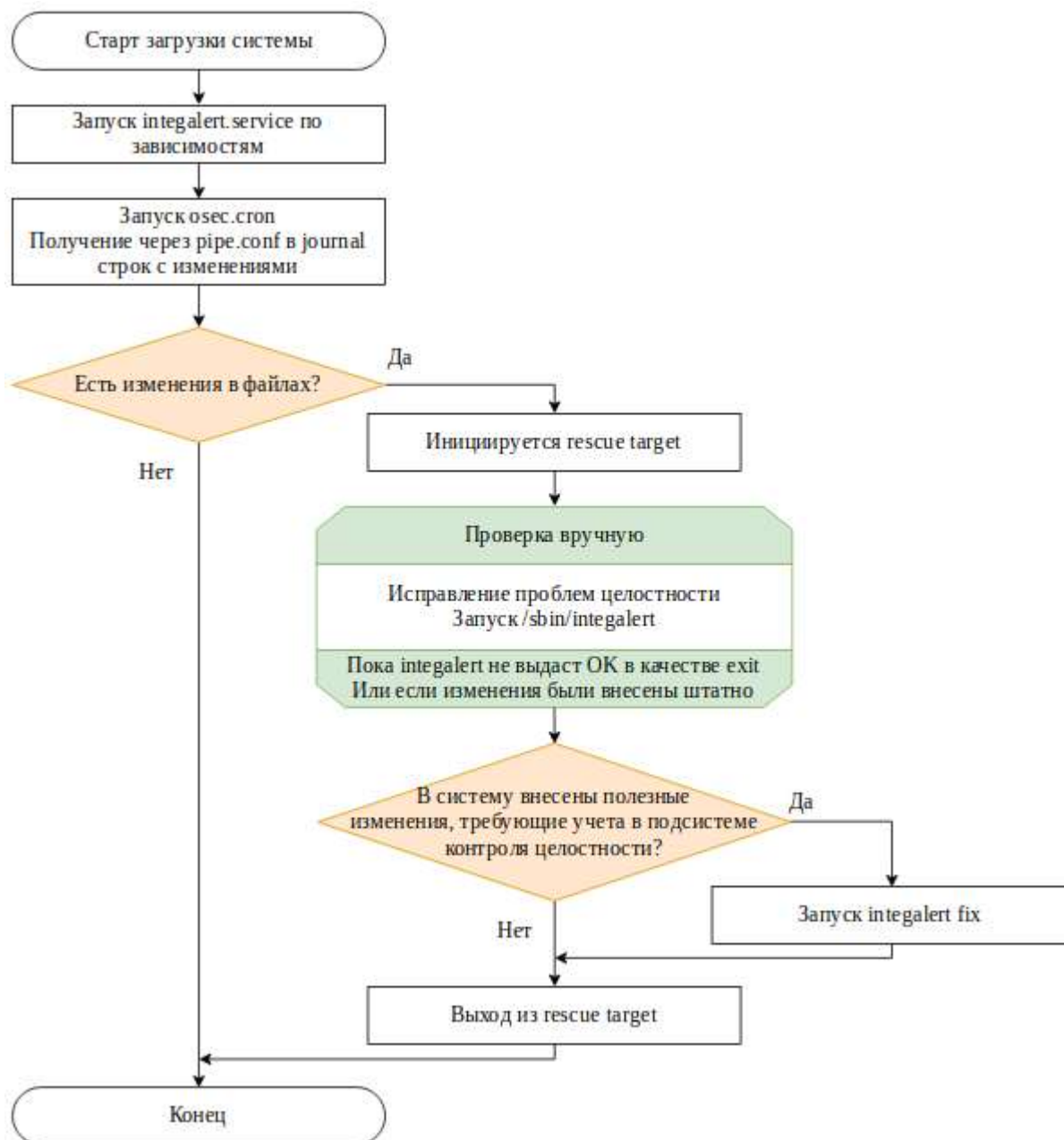
Рис. 6 – Схема проверки целостности при загрузке системы
