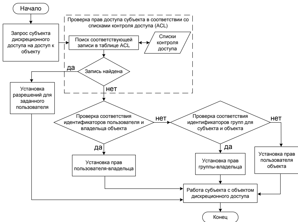
Рис. 3 – Алгоритм функционирования модели дискреционного управления доступом
