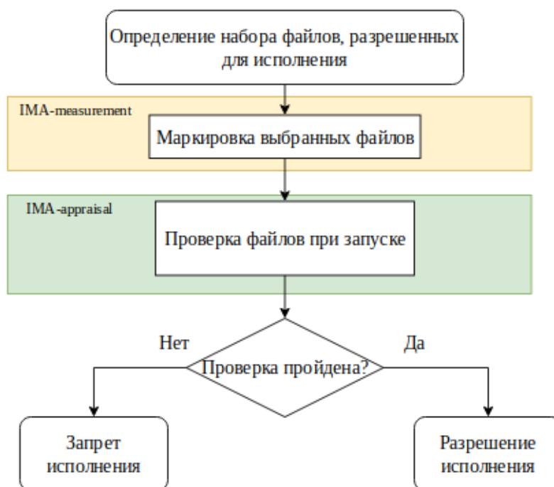
Рис. 4 – Схема функционирования
