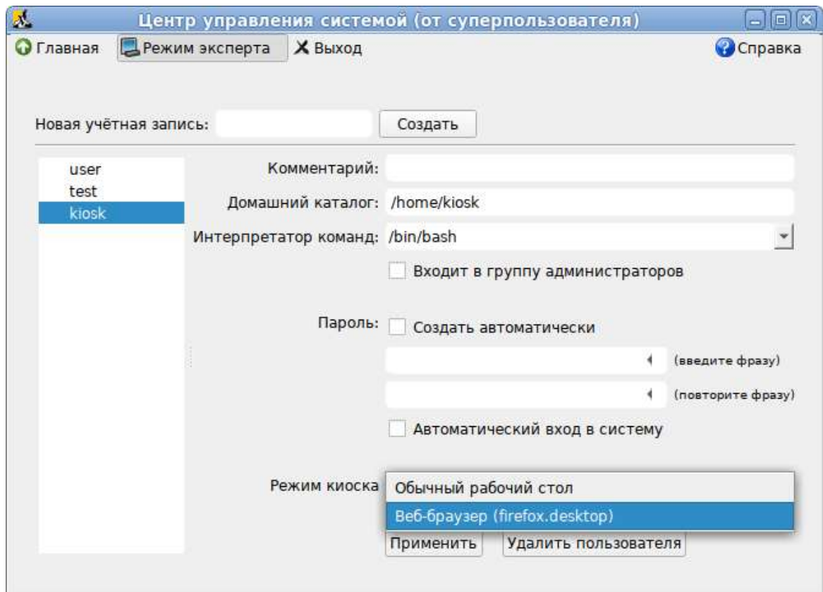
Рис. 11 – Настройка режима «киоск» для пользователя kiosk
