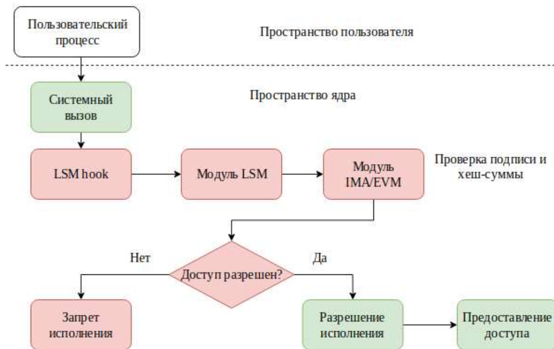
Рис. 5 – Перехват системного вызова и передача управления модулям безопасности
