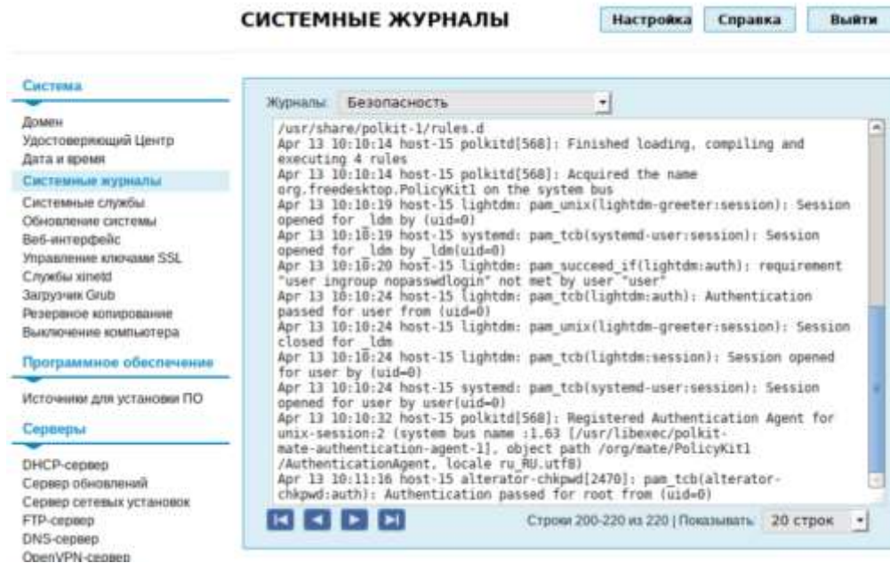
Рис. 16 – Веб-интерфейс просмотра системных журналов
