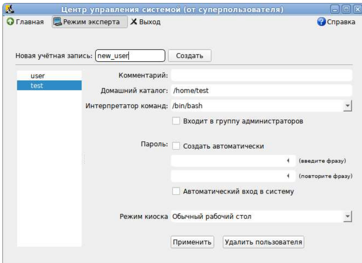
Рис. 9 – Управление локальными пользователями в графическом интерфейсе ЦУС
