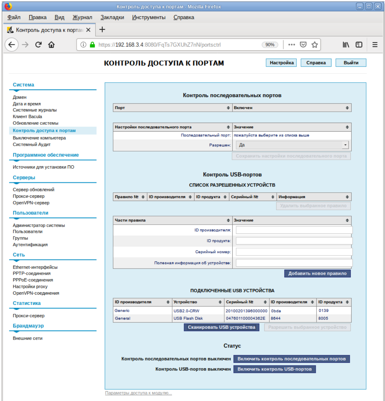
Рис. 12 – Контроль доступа к портам
